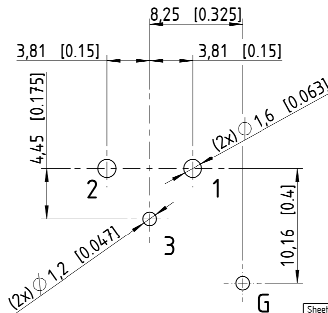
Print-Bohrplan (Bestückungsseite) PCB-Layout (component side)
